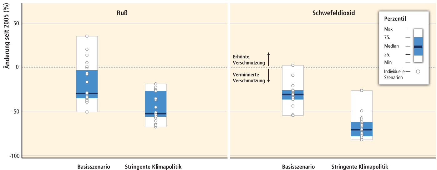
Abbildung SPM.6 Emissionsniveaus für die Luftschadstoffe Ruß und Schwefeldioxid ( \text{SO}_2 ) im Jahr 2050 gegenüber 2005 (0 = Niveau von 2005). Basisszenarien ohne zusätzliche Bemühungen zur Verringerung von THG-Emissionen über die heute bestehenden hinaus werden mit Szenarien mit ambitionierten Minderungsmaßnahmen verglichen, die mit dem Erreichen von ca. 450 bis ca. 500 (430–530) ppm \text{CO}_2 -Konzentrationen bis zum Jahr 2100 vereinbar sind. [Abbildung 6.33]
