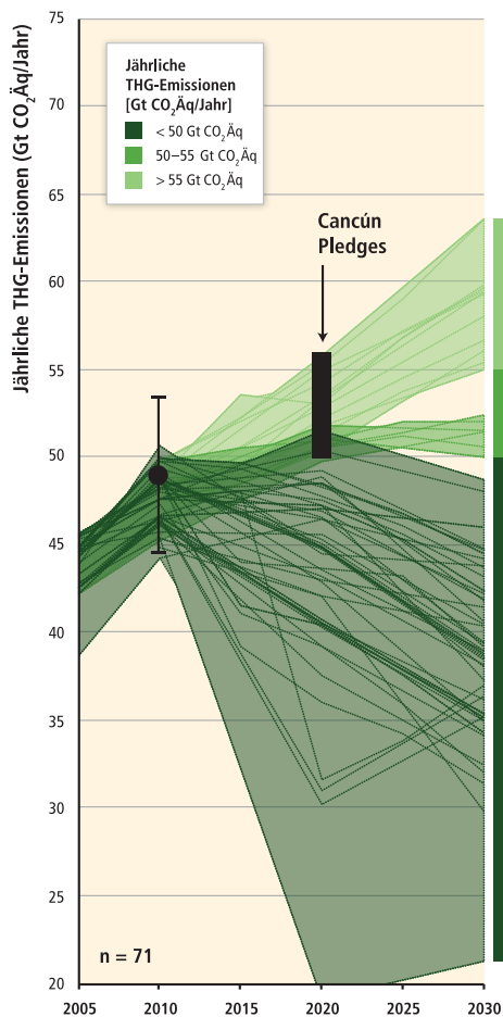
THG-Emissionspfade bis 2030
