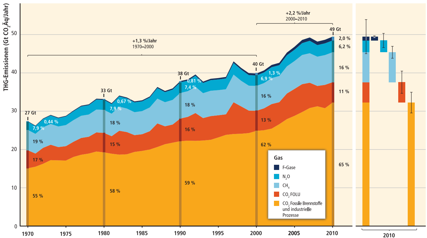
Gesamte jährliche anthropogene THG-Emissionen nach Gruppen von Gasen 1970–2010:
