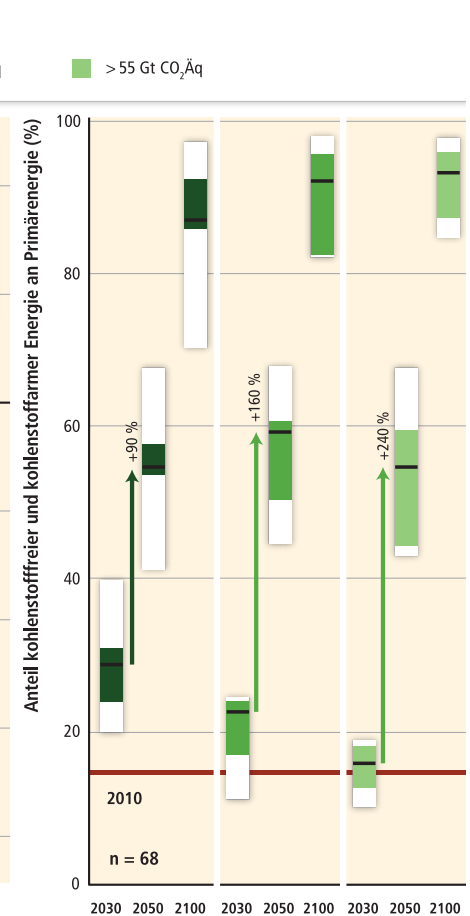
Auswirkungen unterschiedlicher THG-Emissionsniveaus in 2030 auf den Ausbau kohlenstoffarmer Energie
