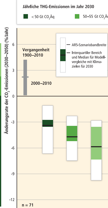
Auswirkungen unterschiedlicher THG-Emissionsniveaus in 2030 auf die jährliche durchschnittliche CO 2 -Emissionsminderungsrate von 2030–2050
