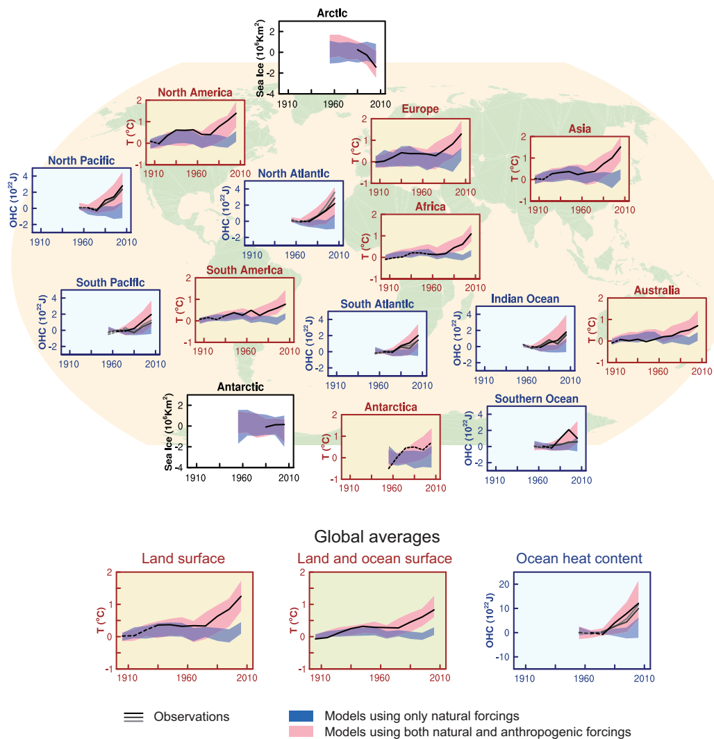
Figuur SPM. 6. Vergelijking van waargenomen en gemodelleerde klimaatverandering voor drie grootschalige indicatoren in de atmosfeer, cryosfeer en de oceaan: verandering in de temperatuur boven land nabij het aardoppervlak (gele panelen), zeeijs in het noordpool- en zuidpoolgebied (witte panelen), en opname van warmte door het bovenste deel van de oceaan (blauwe panelen). Wereldwijd gemiddelde veranderingen zijn ook weergegeven. Alle tijdseries zijn tien jaar-gemiddelden, weergegeven voor het midden van de 10 jaar periode. De zwarte lijnen tonen de waargenomen temperatuur en zijn gestreept als in minder dan 50% van de beschouwde gebieden metingen beschikbaar zijn. Bij de opname van warmte door de oceaan en bij zeeijs betekent een doorgetrokken lijn dat de beschikbaarheid van metingen op z'n minst goed is, en een gestreepte lijn dat de beschikbaarheid slechts redelijk is en dus de onzekerheid groter is. Modelresultaten zijn weergegeven als gemiddelde van de CMIP5 modellen, waarbij de gekleurde band het 5-95% betrouwbaarheidsinterval weergeeft. De blauwe lijn geeft de gemodelleerde klimaatverandering door natuurlijke oorzaken, de rode lijn die door natuurlijke plus menselijke oorzaken.
