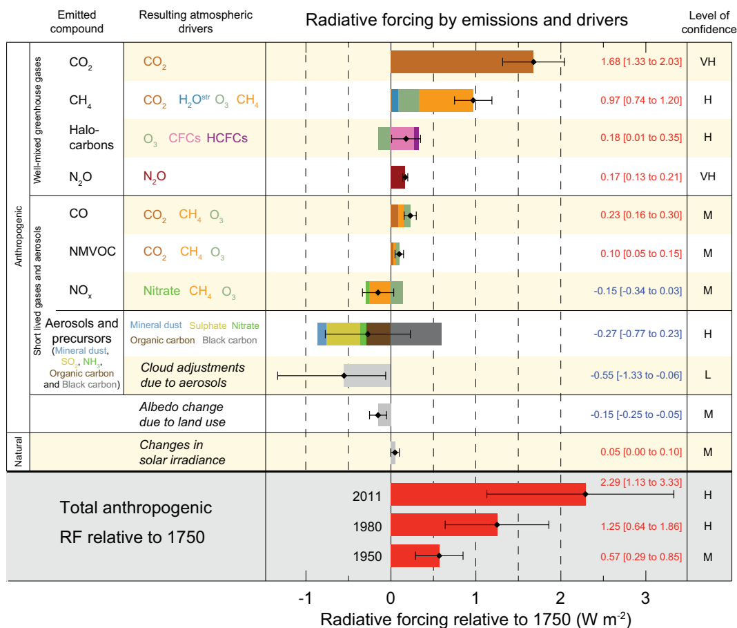
Figuur SPM. 5. De wereldwijd gemiddelde stralingsforcering in 2011 ten opzichte van 1750 voor de belangrijkste oorzaken van klimaatverandering, inclusief de onzekerheden daarin. De beste schatting van de stralingsforcering is aangegeven met een zwarte ruit met bijbehorende onzekerheidsinterval; de numerieke waarden zijn weergegeven rechts in de figuur, samen met de mate van zekerheid (VH - zeer hoog, H - hoog, M - redelijk, L - laag, VL - zeer laag). Kleine forceringen door vliegtuigsporen, HFCs, PFCs en SF 6 zijn niet weergegeven. De totale stralingsforcering door menselijke toedoen sinds 1750 is weergegeven voor drie verschillende jaren.
