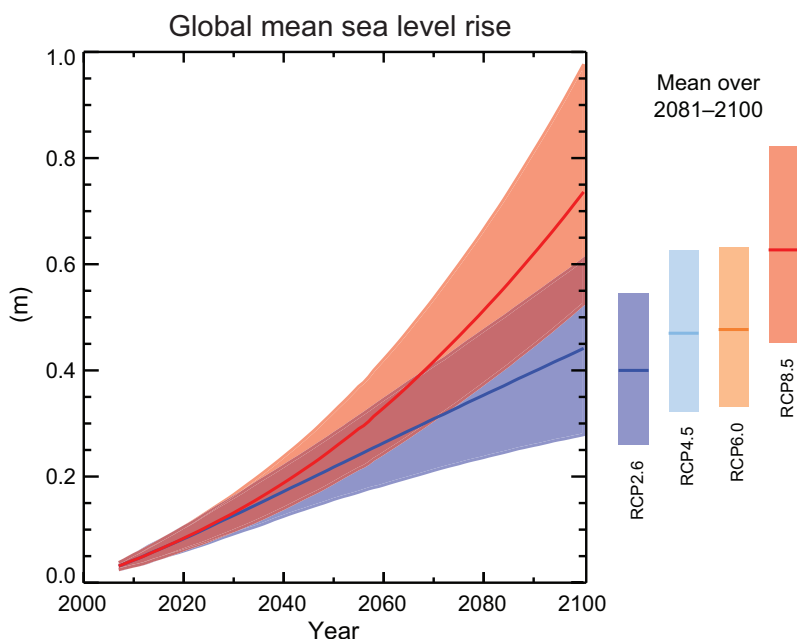
Figuur SPM.9 | Projecties van de wereldwijd gemiddelde zeespiegelstijging in de 21 ste eeuw, ten opzichte van 1986–2005, bepaald uit een combinatie van CMIP5- en zeespiegelmodellen, for de scenario's RCP2.6 en RCP8.5. De waarschijnlijke onzekerheidsmarge is weergegeven met een gekleurde band. De mediane waarden en waarschijnlijke onzekerheidsmarges voor alle RCP-scenario's voor de periode 2081–2100 zijn weergegeven rechts in de figuur. {table 13.5, figure 13.10 en 13.11, Figure TS.21 en TS.22}
