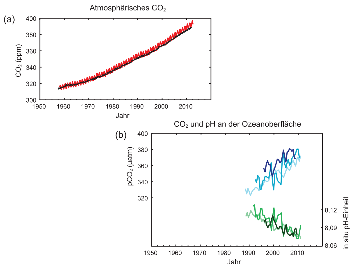
Abbildung SPM.4 | Mehrfache beobachtete Indikatoren eines sich verändernden globalen Kohlenstoffkreislaufs: (a) Atmosphärische Kohlendioxid ( \text{CO}_2 )-Konzentrationen vom Mauna Loa ( 19^\circ 32' \text{N} , 155^\circ 34' \text{W} – rot) und vom Südpol ( 89^\circ 59' \text{S} , 24^\circ 48' \text{W} – schwarz) seit 1958. (b) Teildruck von gelöstem \text{CO}_2 an der Ozeanoberfläche (blaue Kurven) und in situ pH (grüne Kurven), ein Maß für den Säuregehalt des Ozeanwassers. Die Messungen stammen von drei Stationen aus dem Atlantik ( 29^\circ 10' \text{N} , 15^\circ 30' \text{W} – dunkelblau/dunkelgrün; 31^\circ 40' \text{N} , 64^\circ 10' \text{W} – blau/grün) und dem Pazifischen Ozean ( 22^\circ 45' \text{N} , 158^\circ 00' \text{W} – hellblau/hellgrün). Vollständige Einzelheiten der hier dargestellten Datensätze sind im zugrundeliegenden Bericht und im Zusatzmaterial zur Technischen Zusammenfassung zu finden. (Abbildungen 2.1 und 3.18; Abbildung TS.5)
