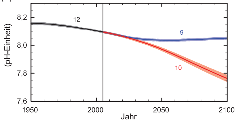
Abbildung SPM.7 | CMIP5 Multimodell-simulierte Zeitreihen von 1950 bis 2100 für (a) die Änderung der mittleren globalen Erdoberflächentemperatur bezogen auf 1986–2005, (b) Ausdehnung des nordhemisphärischen Meereises im September (gleitendes 5-Jahres-Mittel), und (c) mittlerer globaler pH an der Meeresoberfläche. Die Zeitreihen der Projektionen und ein Maß für die Unsicherheit (Schattierung) sind für die Szenarien RCP2.6 (blau) und RCP8.5 (rot) dargestellt. Schwarz (graue Schattierung) ist die modellierte historische Entwicklung hergeleitet aus historischen rekonstruierten Antrieben. Die über den Zeitraum 2081–2100 berechneten Mittel und die zugehörigen Unsicherheitsbereiche sind für alle RCP-Szenarien als farbige vertikale Balken dargestellt. Die Zahl der für die Berechnung des Multimodell-Mittels verwendeten CMIP5-Modelle ist angegeben. Für die Ausdehnung des Meereises (b) sind das projizierte Mittel sowie die Unsicherheit (Minimum-Maximum-Bereich) nur für den Teilsatz von Modellen dargestellt, die den klimatologischen mittleren Zustand und den Trend des arktischen Meereises von 1979 bis 2012 am genauesten reproduzieren (die Zahl der Modelle ist in Klammern angeführt). Der Vollständigkeit wegen ist das CMIP5-Multimodell-Mittel mit gepunkteten Linien angezeigt. Die gestrichelte Linie stellt nahezu eisfreie Bedingungen dar (d. h. wenn die Ausdehnung des Meereises über mindestens fünf aufeinanderfolgende Jahre weniger als 10^6 \text{ km}^2 beträgt). Für weitere technische Details siehe Zusatzmaterial der Technischen Zusammenfassung. {Abbildungen 6.28, 12.5 und 12.28–12.31; Abbildungen TS.15, TS.17 und TS.20}
