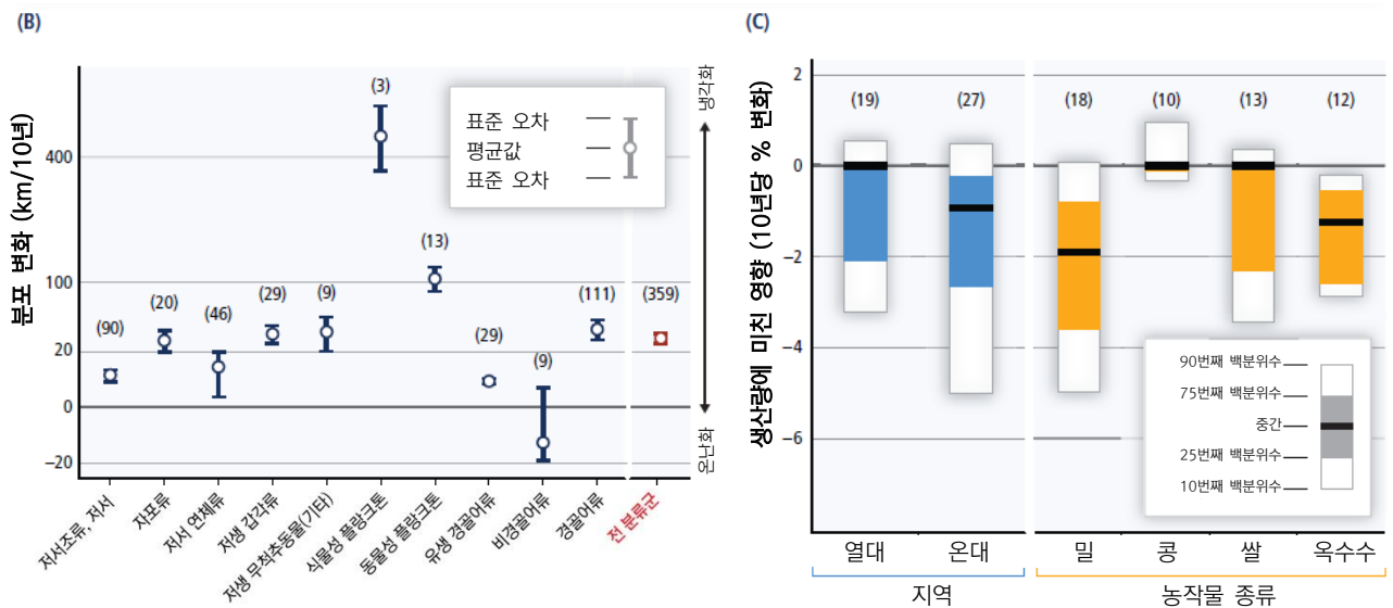
그림 SPM. 2 | 지속적으로 변화하는 세계에서 나타난 광범위한 영향. (A) 최근 수십 년간 기후변화에 의해 발생한 영향의 전 지구적 경향 (AR4 이후의 연구 기반). 전 세계 지도 위에 지리적 분류에 따라 표시하였으며, 각 기호(symbol)들은 해당 영향에 대한 원인이 기후변화로 규명된 것의 범주(카테고리)를 나타낸다. 이와 더불어 관측된 영향에 대한 기후변화의 상대적 기여도 (중요한 또는 덜 중요한)와 규명된 원인에 대한 신뢰도 또한 표시하였다. 영향에 대한 자세한 설명은 보충 표 SPM. A1을 참조한다. (B) 1900 - 2010년에 관측된 해양 분류군 분포 변화의 평균속도 (km/10년). 양수 값의 분포 변화(positive distribution changes)는 온난화와 일치한다 (일반적으로 이전에 더 한류였던 곳 과 극 방향으로 이동). 각 범주마다 분석 분류군의 수를 괄호 안에 표기하였다. (C) 1960 - 2013년에 걸쳐, 관측된 기후변화가 온대 및 열대 지방의 4 가지 주요 농작물 수확량에 미쳤을 것으로 추정되는 영향 요약. 각 범주마다 분석 지점의 수를 괄호 안에 표시하였다. [그림 7-2, 18-3 및 MB-2]
