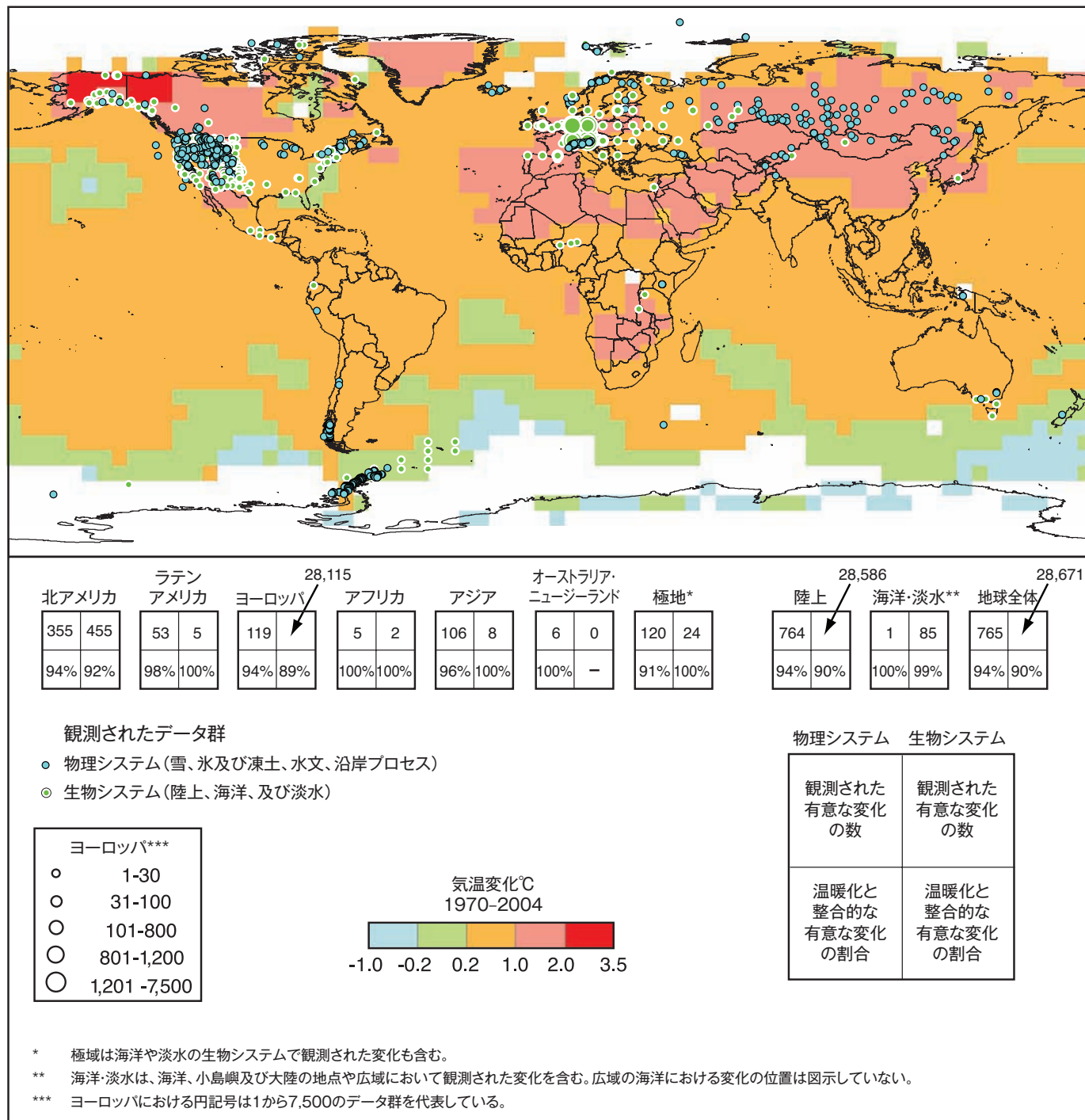
図 SPM.1. この図は、物理システム (雪氷、凍土、水文及び沿岸プロセス) 及び生物システム (陸域、海洋及び淡水の生物システム) のデータ群における有意な変化があった地点を、1970年から2004年の間における地上気温の変化とともに示している。577の研究による約80,000件のデータ群から約29,000件のデータ群が選ばれた。これらは、以下の基準に合致するものである：(1) 1990年かそれ以降まで続く；(2) 少なくとも20年間は継続している；(3) 各研究における評価で、いずれかの方向に有意な変化を示している。これらのデータは約75の研究 (うち約70件は第3次評価報告書以降の新しい研究) から引用されており、約29,000件のデータ群を含み、うち約28,000件はヨーロッパの研究によるものである。空白で示された地域は、気温のトレンドを推定するに足るだけの気候観測データを有していない。2×2ます目のボックスでは、有意な変化を示したデータ群の総数 (上列) とそれらのうち温暖化と整合するものの割合 (下列) を以下の地域について示している、(i) 大陸域：北アメリカ、ラテンアメリカ、ヨーロッパ、アフリカ、アジア、オーストラリア・ニュージーランド、及び極域、(ii) 地球規模：陸域、海洋・淡水、及び地球全体。7つの地域ボックスの研究数の合計は、地球全体の数に満たないが、これは極域以外の地域の数には海洋・淡水システムに関するものが含まれていないためである。広域にわたる海洋変化の地点は地図上には示されていない [第2作業部会第4次評価報告書 図1.8, 図1.9; 第1作業部会第4次評価報告書 図3.9b]。
