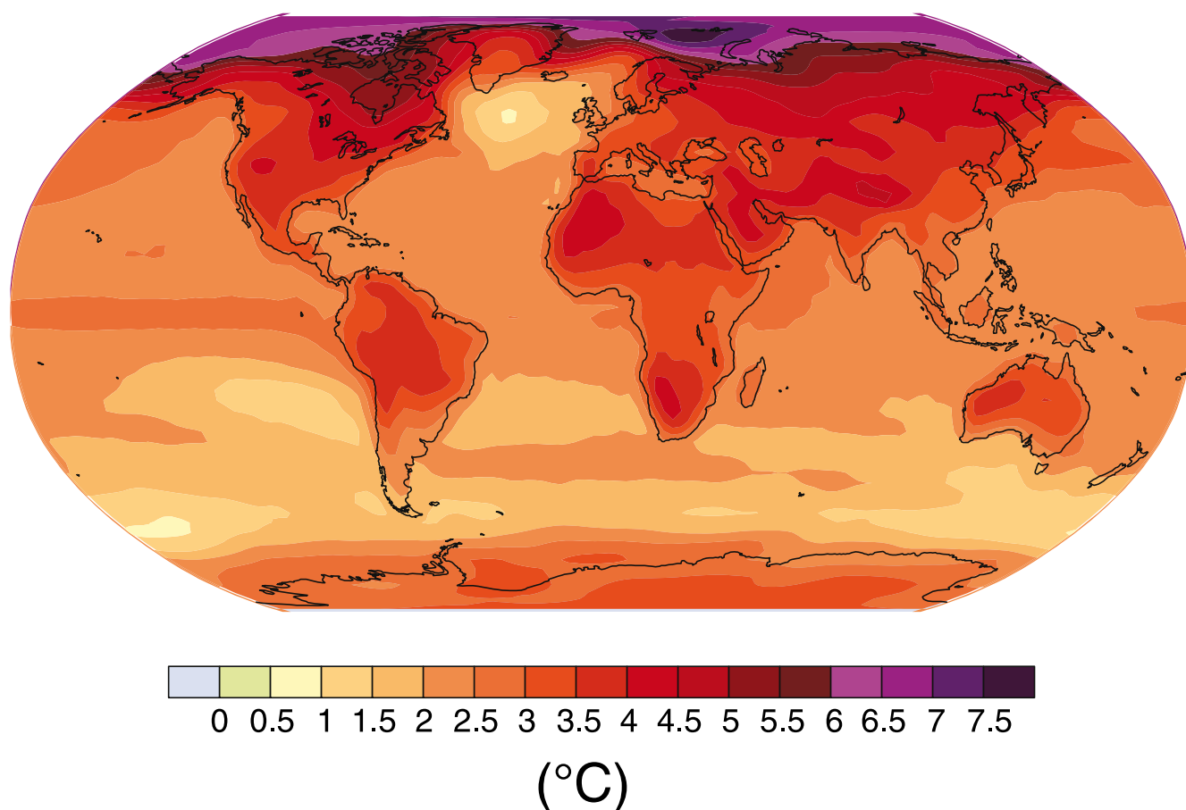
Figur SPM 6. Projektioner över förändringar av jordytans temperatur för slutet av 2000-talet (2090–2099). Kartan visar genomsnittsprojektioner enligt AOGCM för SRES-scenariet A1B. Alla temperaturer anges relativt perioden 1980–1999. {Figur 3.2}
