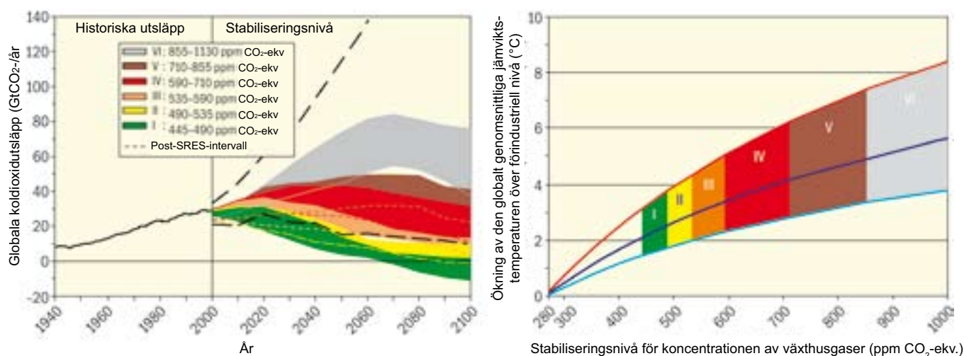
Figur SPM 11. Globala koldioxidutsläpp för perioden 1940–2000 och utsläppsintervall för olika kategorier av stabiliseringsscenarier mellan 2000 och 2100 (vänstra bilden); samt motsvarande förhållande mellan stabiliseringsmål och den sannolika globalt genomsnittliga ökningen av jämviktstemperaturen över förindustriell nivå (högra bilden). Det kan ta flera hundra år innan jämvikt nås, särskilt i scenarier med höga stabiliseringsnivåer. De färgade skuggade fälten visar stabiliseringsscenarierna grupperade enligt de olika målen (stabiliseringskategori I–VI). Den högra bilden visar intervall av globalt genomsnittlig temperaturförändring över förindustriell nivå, med (i) "troligaste värde" på klimatkänslighet på 3°C (svart linje i mitten av det skuggade fältet), (ii) den övre gränsen i sannolikhetsintervallet för klimatkänslighet 4,5°C (röd linje högst upp i det skuggade fältet) (iii) den nedre gränsen i sannolikhetsintervallet för klimatkänslighet 2°C (blå linje längs ner i det skuggade fältet). De svarta streckade linjerna i den vänstra bilden visar utsläppsintervallen i nya referensbanescenarier 44 som publicerats sedan SRES (2000). Stabiliseringsscenariernas utsläppsintervall omfattar både scenarier som enbart inkluderar koldioxidutsläpp och scenarier som inkluderar flera gaser och motsvarar 10:e till 90:e percentilen av hela skalan av scenarier.
