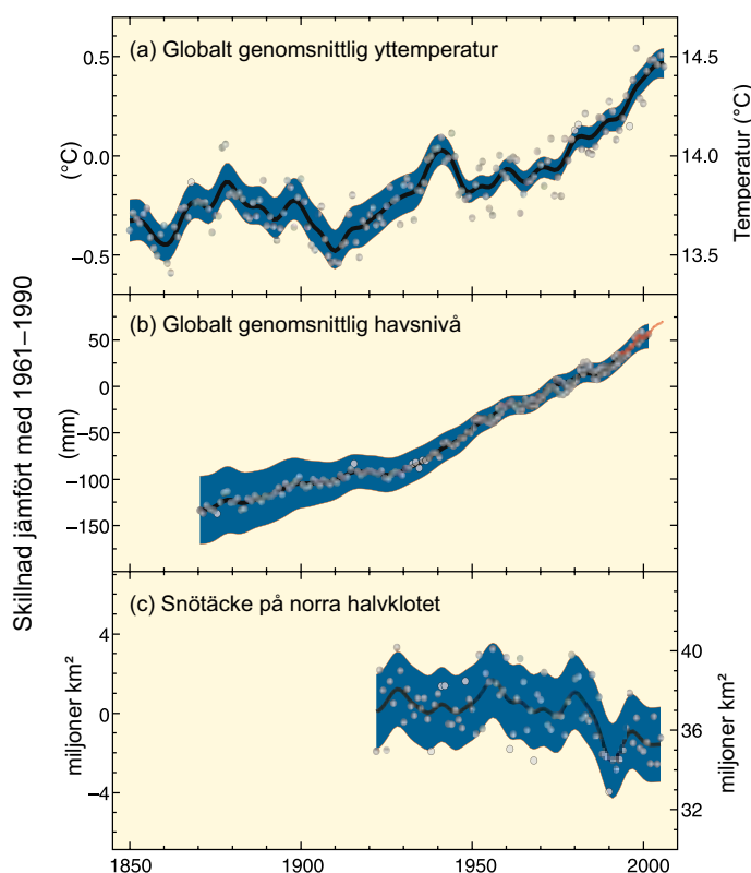
Figur SPM 1. Observerade förändringar av (a) den globalt genomsnittliga ytemperaturen; (b) den globalt genomsnittliga höjningen av havsytanivån enligt mätningar med mareograf 6 (blå) och satellit (röd) samt (c) snötäckets utbredning på norra halvklotet i mars-april. Alla förändringar är i relation till motsvarande genomsnitt för perioden 1961–1990. Utjämnade kurvor representerar genomsnittsvärdet för tioårsperioder medan cirkelarna visar årsgenomsnittet. De skuggade områdena är osäkerhetsintervallen som beräknas utifrån en omfattande analys av kända osäkerhetsfaktorer (a och b) och utifrån tidsserier. {Figur 1.1}
