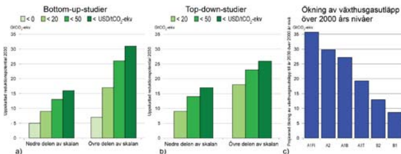
Figur SPM 9. Global ekonomisk reduktionspotential 2030 uppskattad i bottom-up-studier (bild a) och top-down-studier (bild b), jämfört med utsläppsökningen relativt 2000 års utsläpp av växthusgaser på 40,8 GtCO 2 -ekvivalenter enligt projektionerna i SRES-scenarierna (bild c). Anmärkning: För att skapa konsistens med utsläppsresultaten från SRES redovisas utsläppen av växthusgaser 2000 exklusive utsläppen från den förbrukande biomassa ovan jord som återstår efter avverkning och avskogning och emissioner från torvbränder och dränerade torvmossar.
