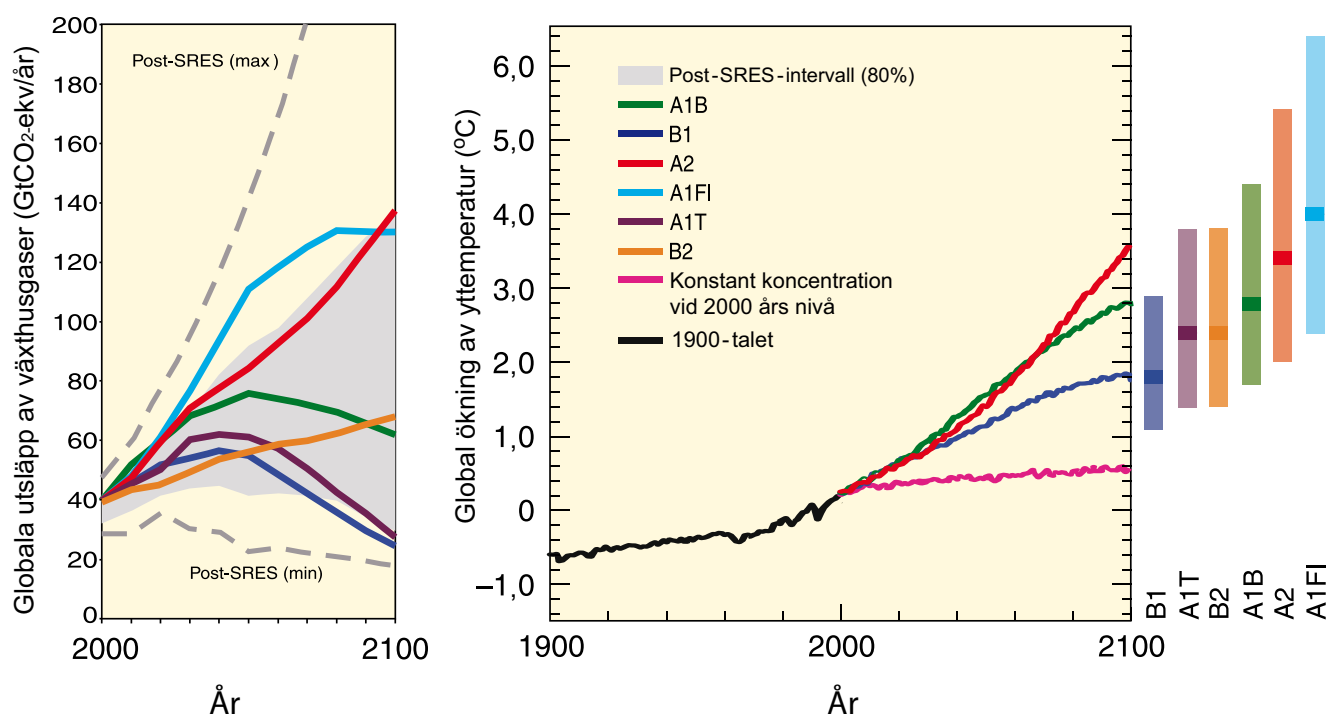
Figur SPM 5. Vänstra bilden: Globala utsläpp av växthusgaser (i CO 2 -ekvivalenter) i frånvaro av klimatpolitiska åtgärder: sex illustrativa markörscenarier ur SRES (färgade linjer) och den 80:e percentilen för senare scenarier som publicerats efter SRES (post-SRES) (gråskuggat fält). De streckade linjerna visar post-SRES-scenariernas fulla vidd. Utsläppen omfattar CO 2 , CH 4 , N 2 O och F-gaser 26 .
