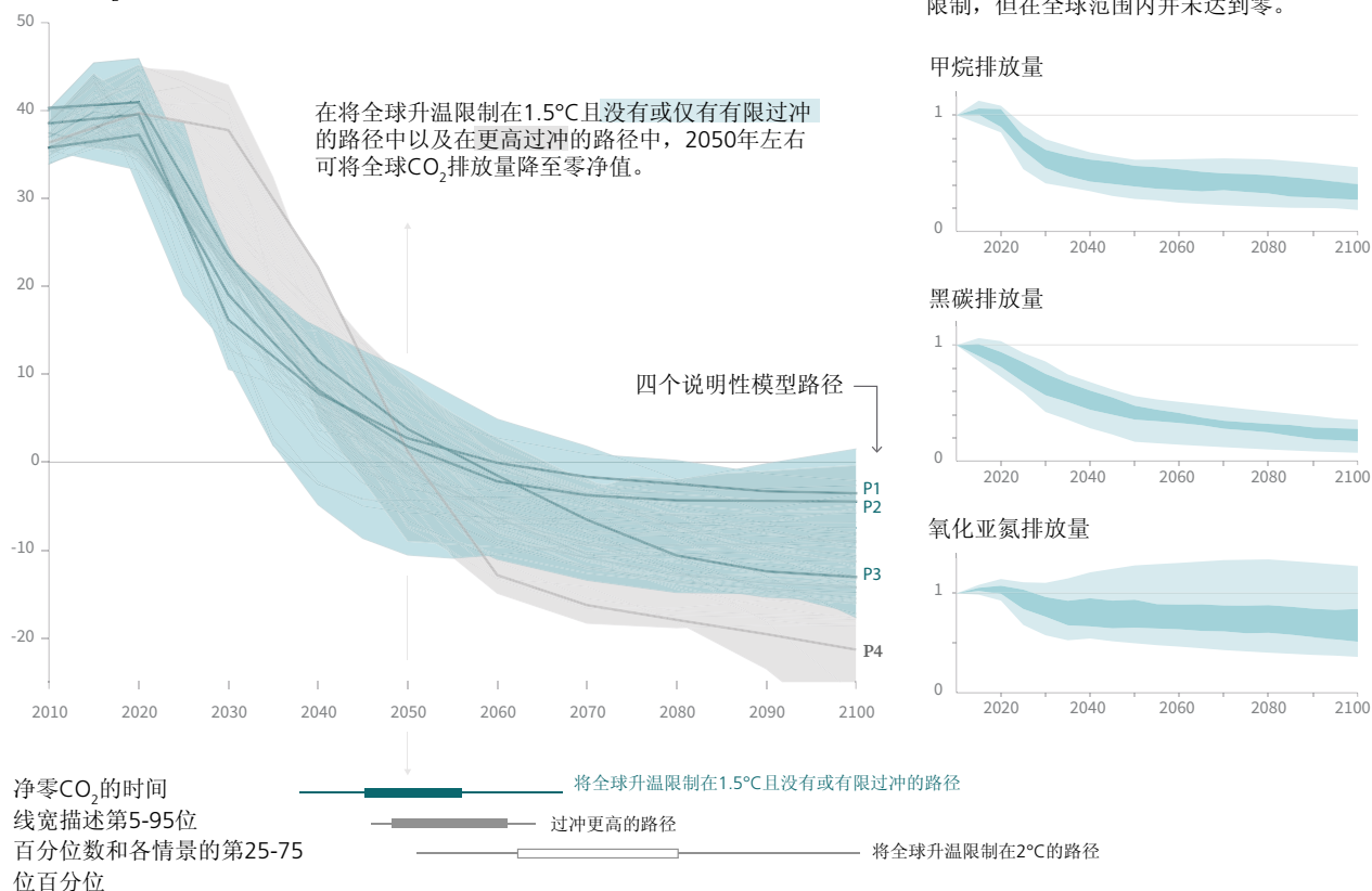
图SPM. 3a: 全球排放途径特征。主图显示在将全球升温限制在1.5°C且没有或仅有限（低于0.1 °C）过冲的路径中，全球净人为CO 2 排放。阴影区显示本报告中分析的全部路径。右图显示了三种具有大量历史强迫的化合物的非CO 2 排放范围，大部分排放来自与CO 2 减缓相关的来源。这些图中的阴影区显示了在将全球升温限制在1.5°C且没有或仅有限过冲的路径中5-95%（浅阴影）和四分位（暗阴影）范围。图底部的盒须图显示了各路径达到全球净零CO 2 排放水平的时间点，并与将全球升温限制在2°C且概率至少为66%的路径进行的比较。四个示例性模型路径在主图中有突出显示，标记为P1、P2、P3和P4，对应于第2章中评估的LED、S1、S2和S5路径。图SPM.3b有这些路径的描述和特征。{2.1, 2.2, 2.3, 图2.5, 图2.10, 图2.11}
